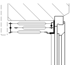
D4 sur cornières à visser 2 faces
