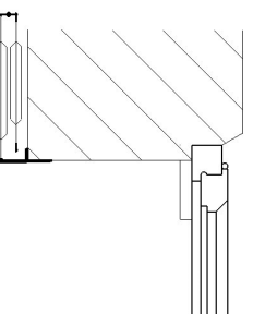
E5 en facade sur cornière d'angle
