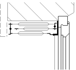
D4 sur cornières à visser 2 faces
