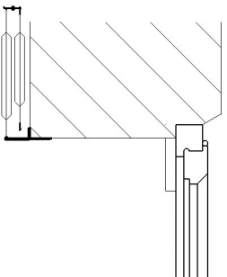
B2 sur tapées bois un vantail en tableau les autres en façade
