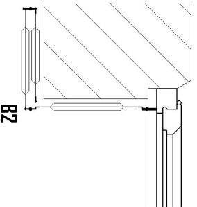
B2 sur tapées bois un vantail en tableau les autres en façade
