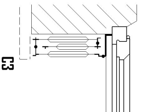
C3 sur tapées cornières petit L intérieur
