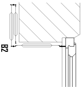
sur tapées bois un vantail en tableau las autres en facade
