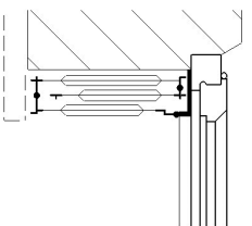
sur cornières à visser 2 faces
