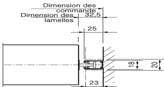
Coulisse simple 25 x18 type 1
