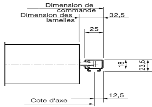
Coulisse simple 25 x18 type 2
