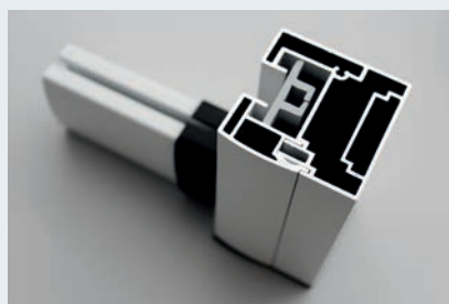
Coulisse en aluminium extrudé laquée
